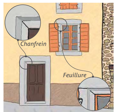
Dessins d'encadrements de baies chanfreinées ( chanfrein* ) et feuillurées. ( ou feuillure* ).
